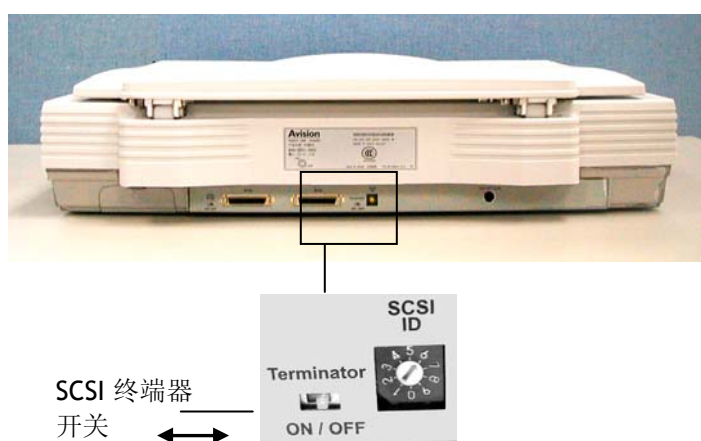
图2-3 SCSI 终端器开关
