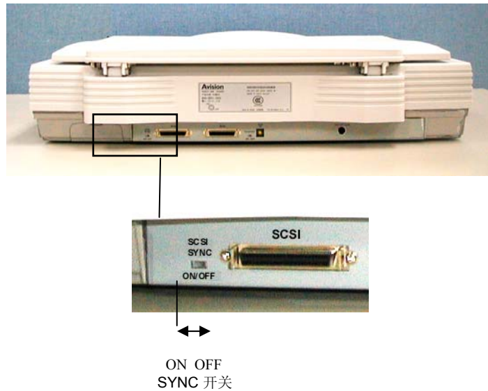
图2-4 SYNC(同步处理) 开关
