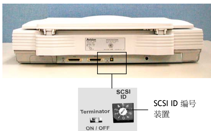
图2-2 SCSI ID 编号设定
